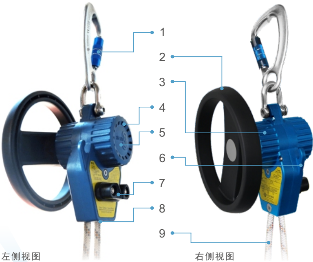
左侧视图
